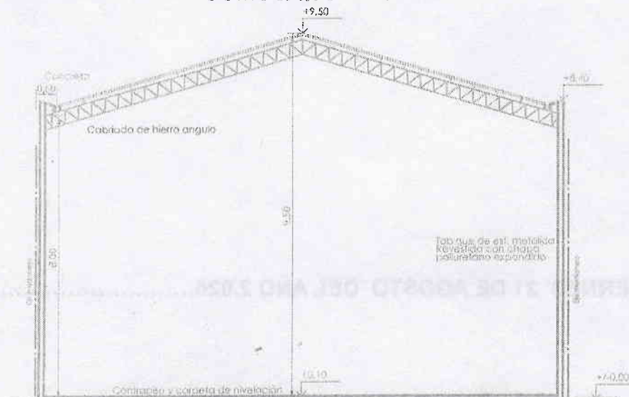
CORTE ESQUEMATICO
