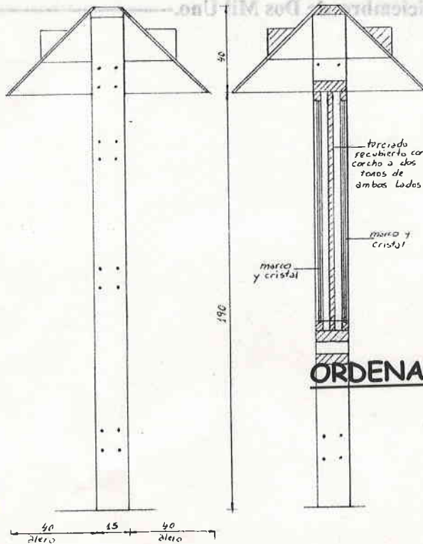
Vistas laterales izq. y der.
