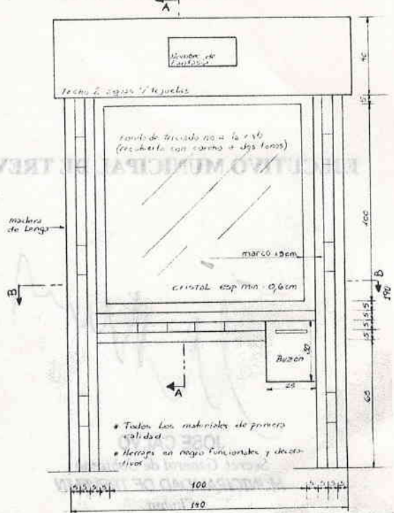
Vistas Fronte y contrafrente
